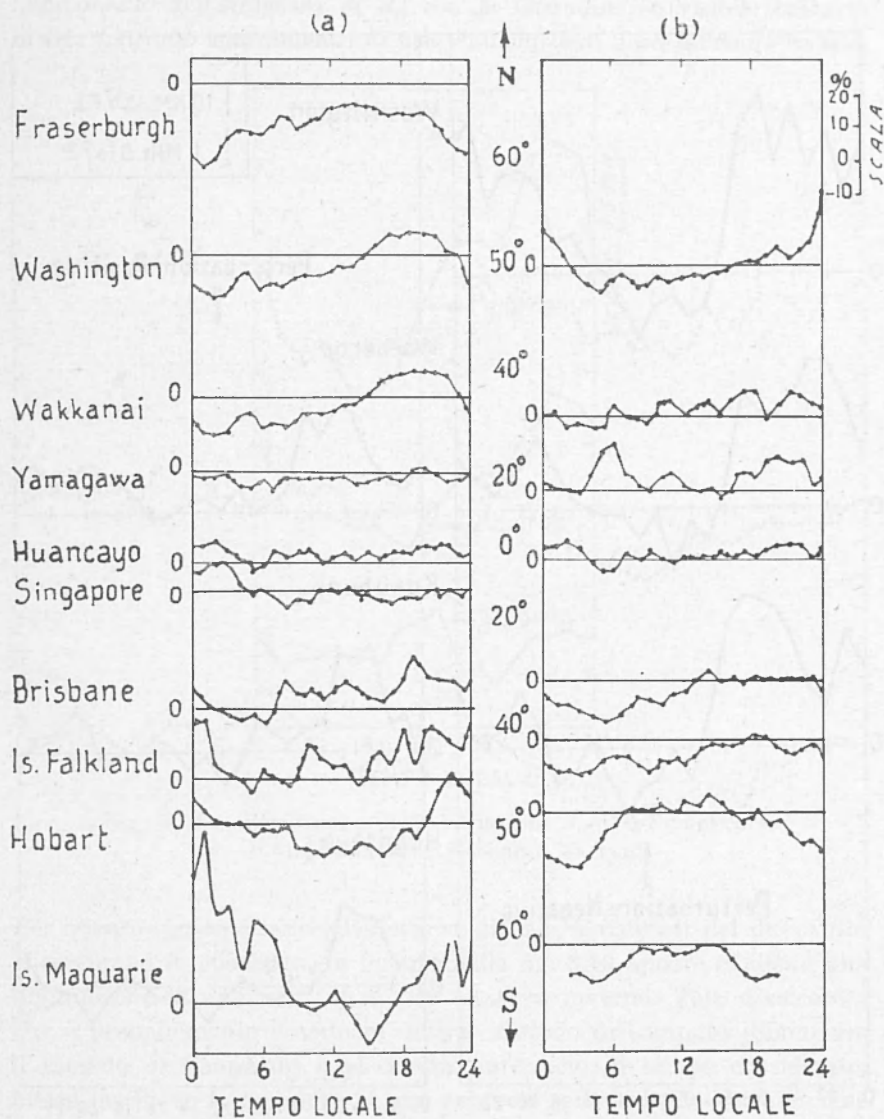
Fig. 3.10 - Variazione S_D di foF2 a varie latitudini: a) estate dell'emisfero nord; b) inverno dell'emisfero nord (secondo Sinno).
