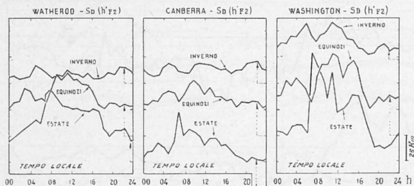
Fig. 3.18 - Effetto stagionale sulla variazione S_D di h'F2 (secondo Martyn).
