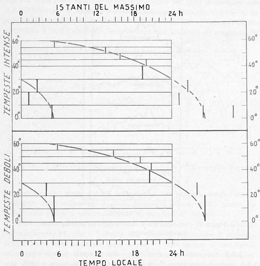
Fig. 3.16 - Distribuzione delle ore (locali) del massimo della componente di 24 ore della variazione S_p di foF2 nelle varie zone di latitudine geomagnetica (secondo Matsushita).
