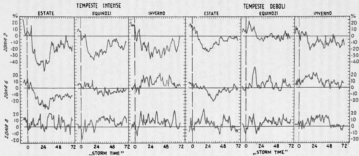
Fig. 3.5 – Effetto stagionale sulla variazione D_{st} di foF2 (secondo Matsushita)
