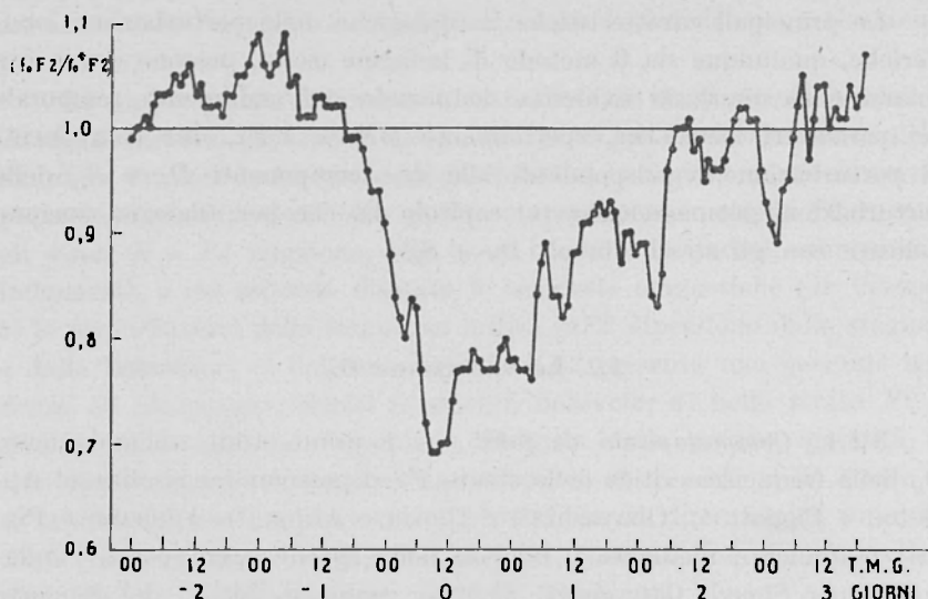
Fig. 3.1 - Andamento medio della variazione relativa di foF2 dal suo valore mediano durante una tempesta ionosferica (secondo Appleton e Piggott).
