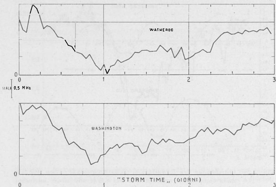
Fig. 3.3 - D_{st} di foF2 a Watheroo (1939-50; 90 tempeste) e a Washington (1941-50; 81 tempeste) (secondo Martyn).
