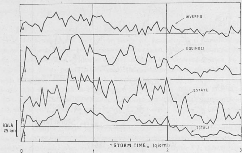
Fig. 3.7 — D_{st} di h'F2 a Watheroo (1939-50) (secondo Martyn).
