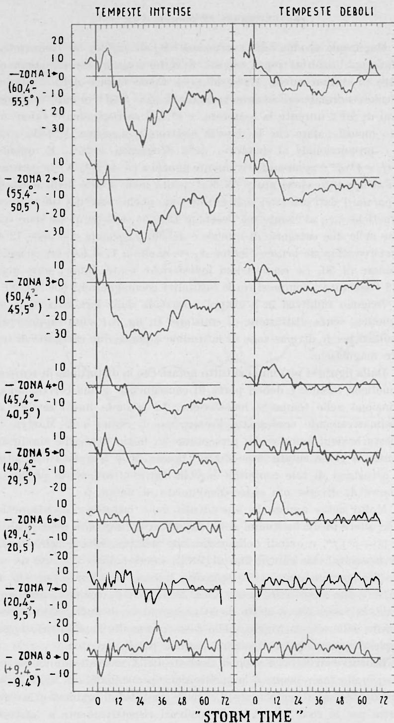
Fig. 3.4 — D_{st} di foF2 per otto zone di latitudine geomagnetica; in ordinate la quantità 200(f-f^*)/f^* (secondo Matsushita).
