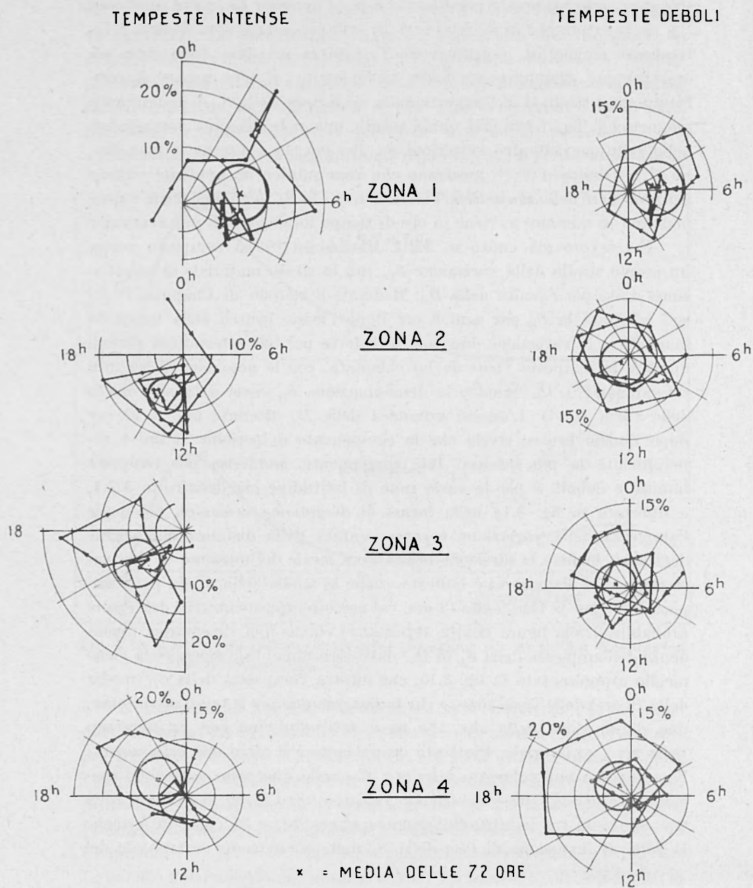
Fig. 3.14 - Diagramma armonico della componente di 24 ore delle variazioni D_5 di foF_2 a varie latitudini (secondo Matsushita).
