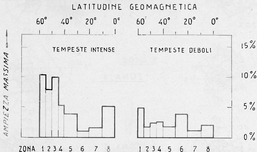
Fig. 3.15 - Distribuzione dell'ampiezza della componente di 24 ore della variazione S_D di foF2 nelle varie zone di latitudine geomagnetica (secondo Matsushita).
