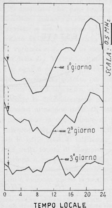
Fig. 3.12 - Evoluzione della variazione S_D di foF2 nel corso di una tempesta (secondo Martyn).
