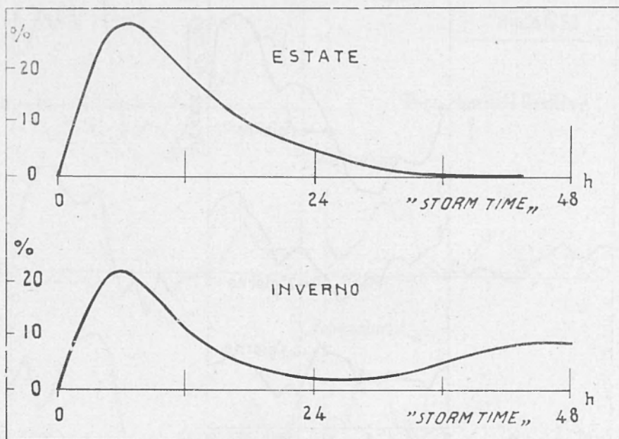
Fig. 3.13 - Sviluppo dell'ampiezza della variazione S_D di foF2 a Washington (1944-51) (secondo Sinno).
