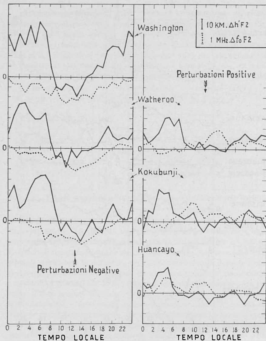
Fig. 3.11 — Variazione S_D di foF2 (-----) e hpF2 (——) a varie latitudini (secondo Sato).
