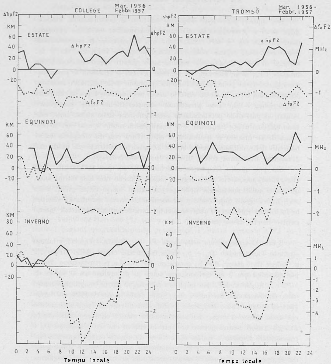
Fig. 3.21 - Variazione S_D di foF2 (-----) e di hpF2 (—) nella zona aurorale (secondo Sato).
