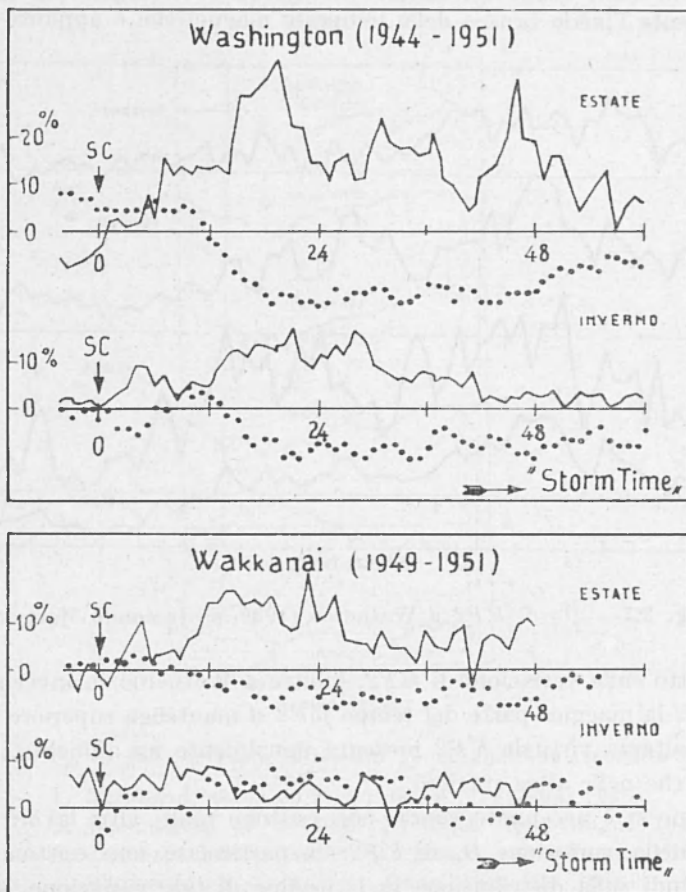
Fig. 3.6 - D_{st} per lo strato F2 a Washington e Wakkanai: ..... foF2 , ——— h'F2 (secondo Sinno).
