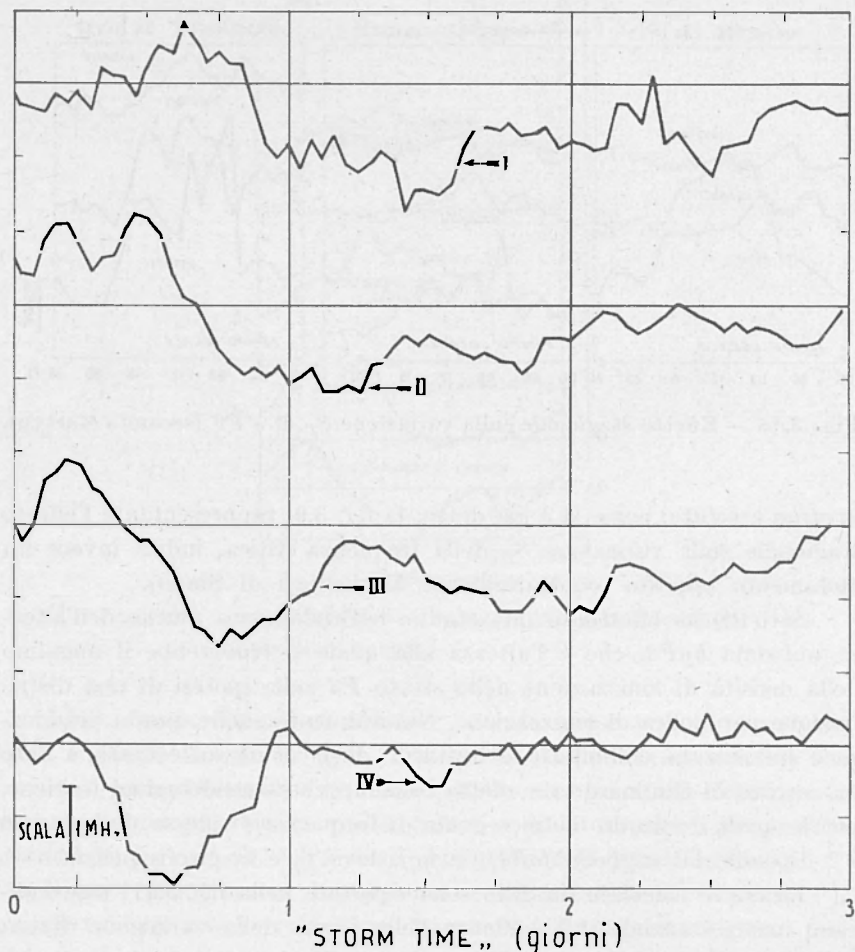
Fig. 3.19 — Variazione di foF_2 a Watheroo per i primi tre giorni di tempeste ionosferiche associate a tempeste magnetiche a inizio brusco. I, inizio brusco tra 2 h e 5 h (tempo locale); II, tra 8 h e 11 h ; III, tra 14 h e 17 h ; IV, tra 20 h e 23 h (secondo Martyn).
