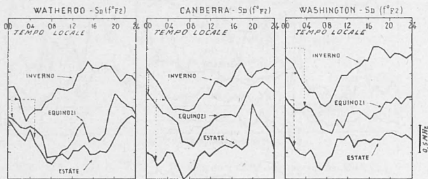
Fig. 3.9 — Effetto stagionale sulla variazione S_D di foF2 (secondo Martyn).
