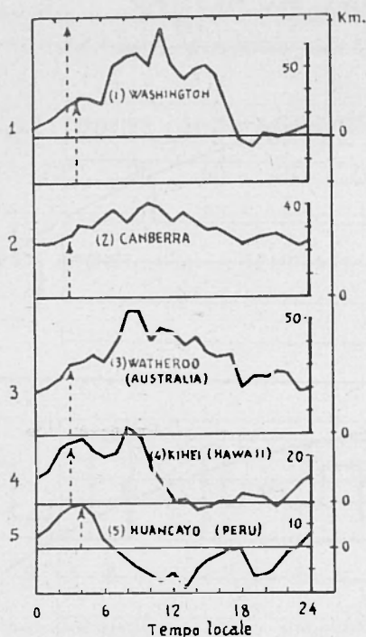
Fig. 3.17 - S_D di h'F2 a varie latitudini geomagnetiche (secondo Martyn).
