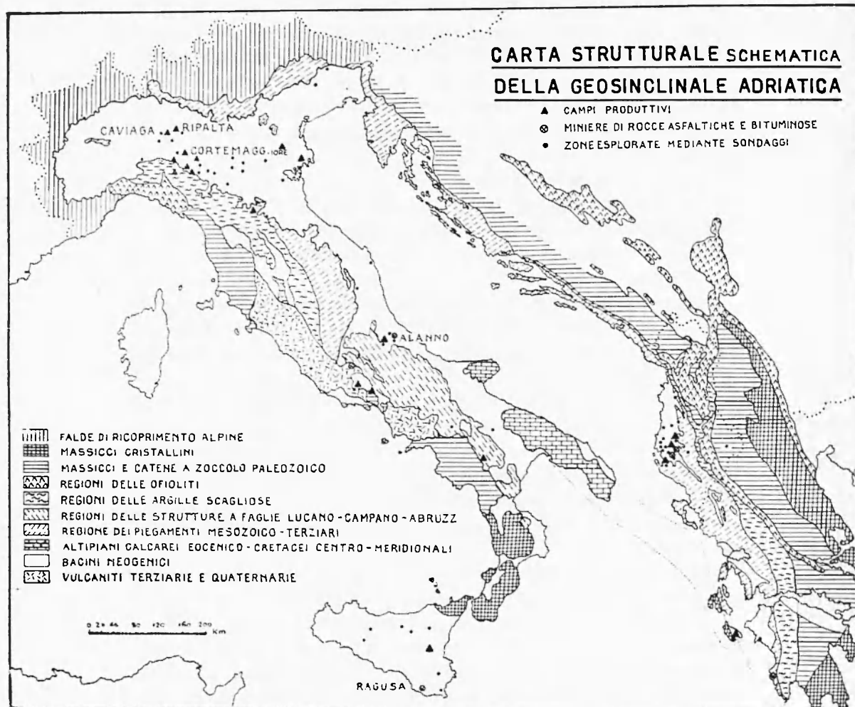
Fig. 5 - Schema strutturale della geosinclinale adriatica (G. Ineichen, 1951).
