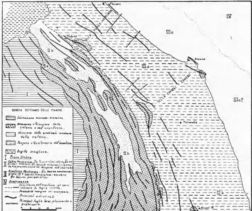
Fig. 7 - Schema tettonico delle Marche, secondo Selli, 1951.
