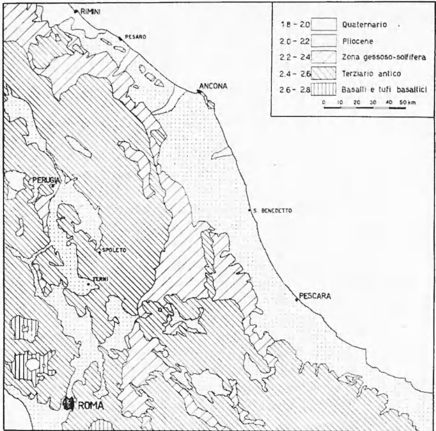
Fig. 3 - Schema della densità media fino al livello del mare, adottata per il calcolo della correzione di Bouguer.
