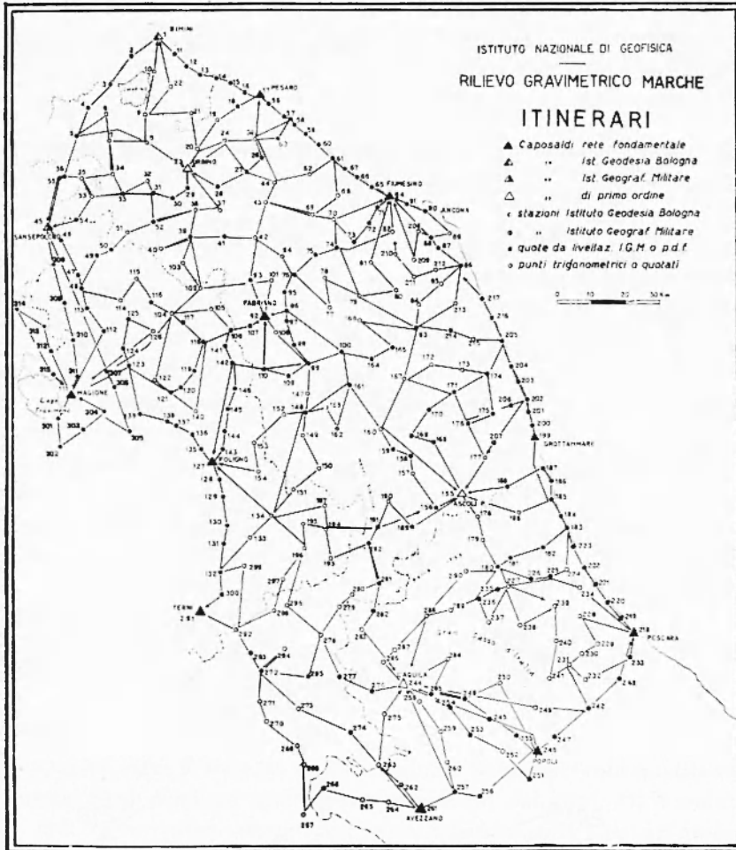
Fig. 1 - Distribuzione delle stazioni gravimetriche, itinerari e ripetizioni.
