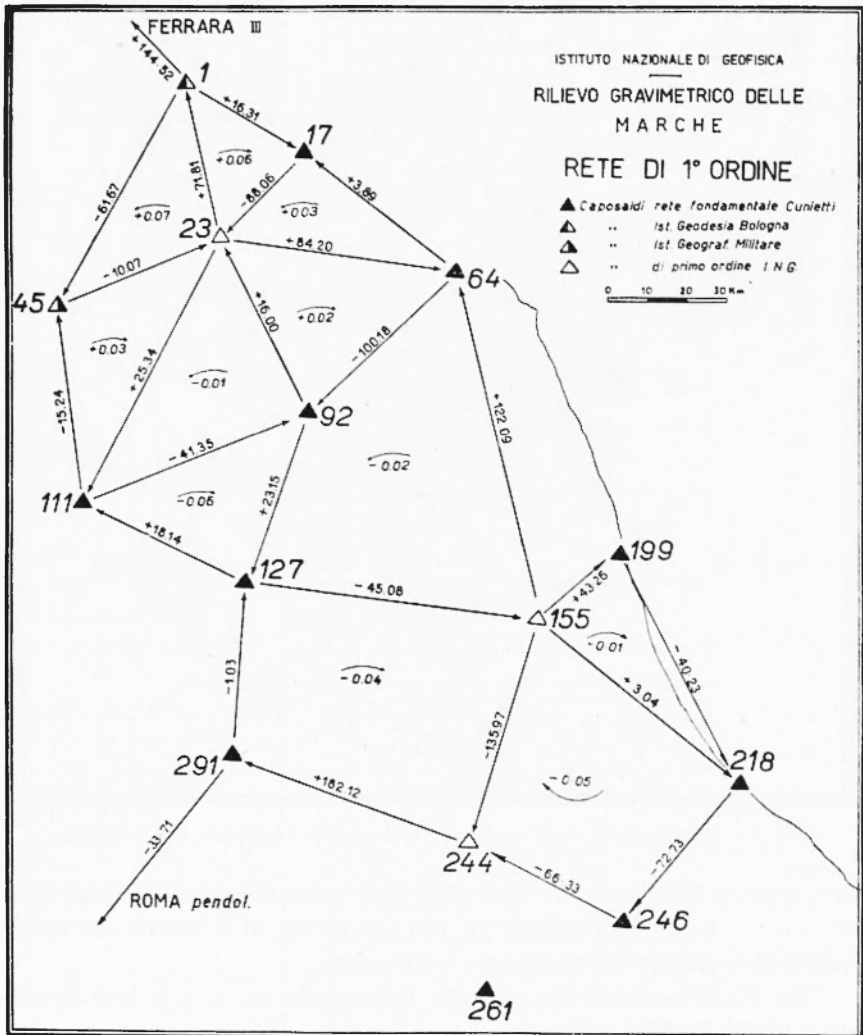
Fig. 2 - Collegamenti fra i caposaldi ed errori di chiusura (in mgal).
