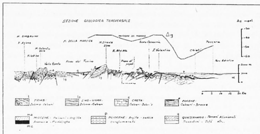
Fig. 9 - Correlazione fra l'anomalia gravimetrica \Delta g e la sezione geologica trasversale secondo Beneo, 1939.
