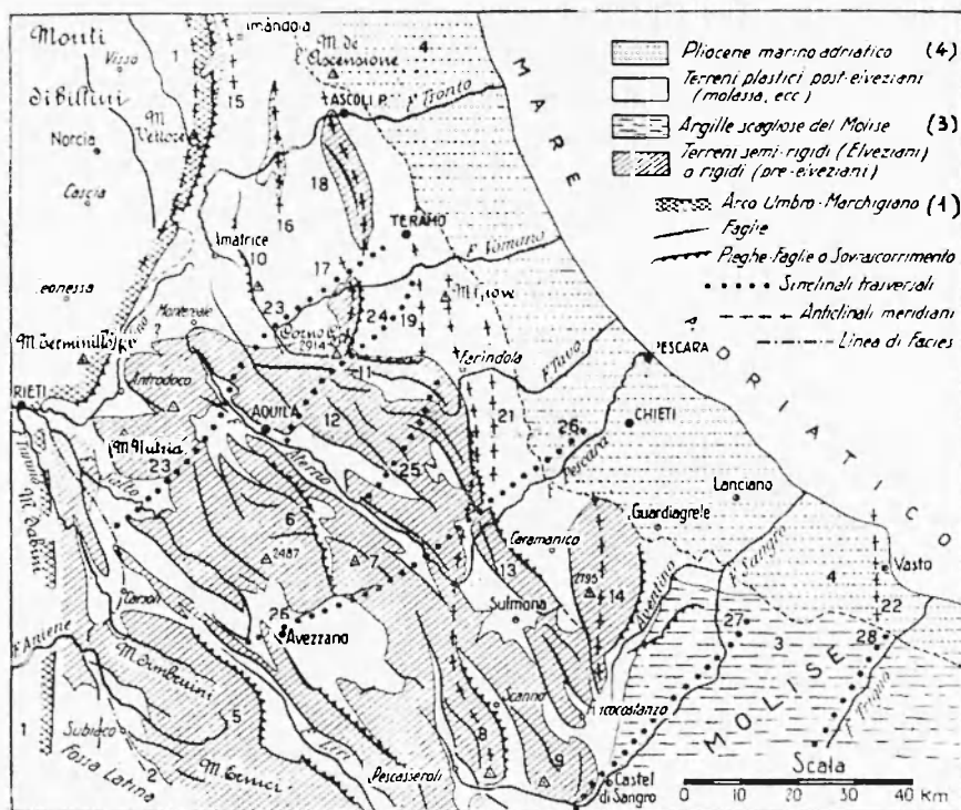
Fig. 8 - Gli assi tettonici dell'Appennino abruzzese, secondo Demangeot, 1952.
