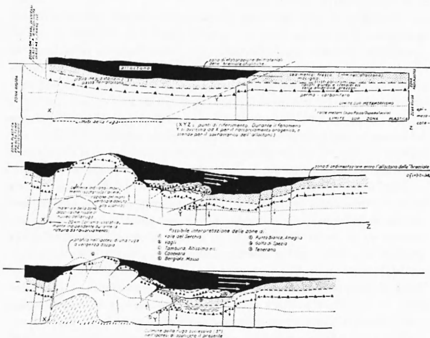
Fig. 6 - Evoluzione di una ruga tettonica, nell'Appennino sett. (secondo Merla, 1951).
