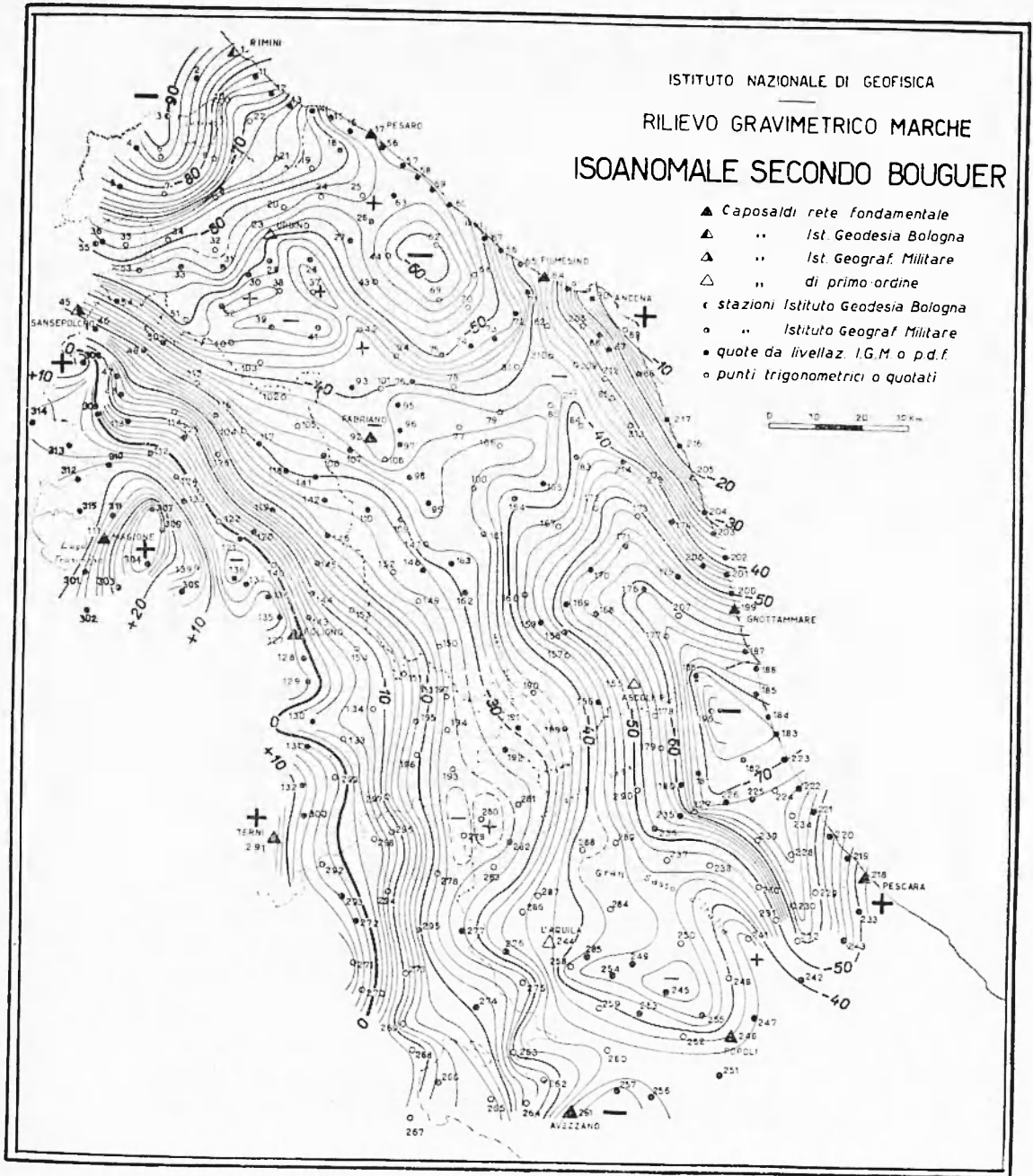
Fig. 4 - Isoanomale secondo Bouguer (equidistanza 2 mgal).
