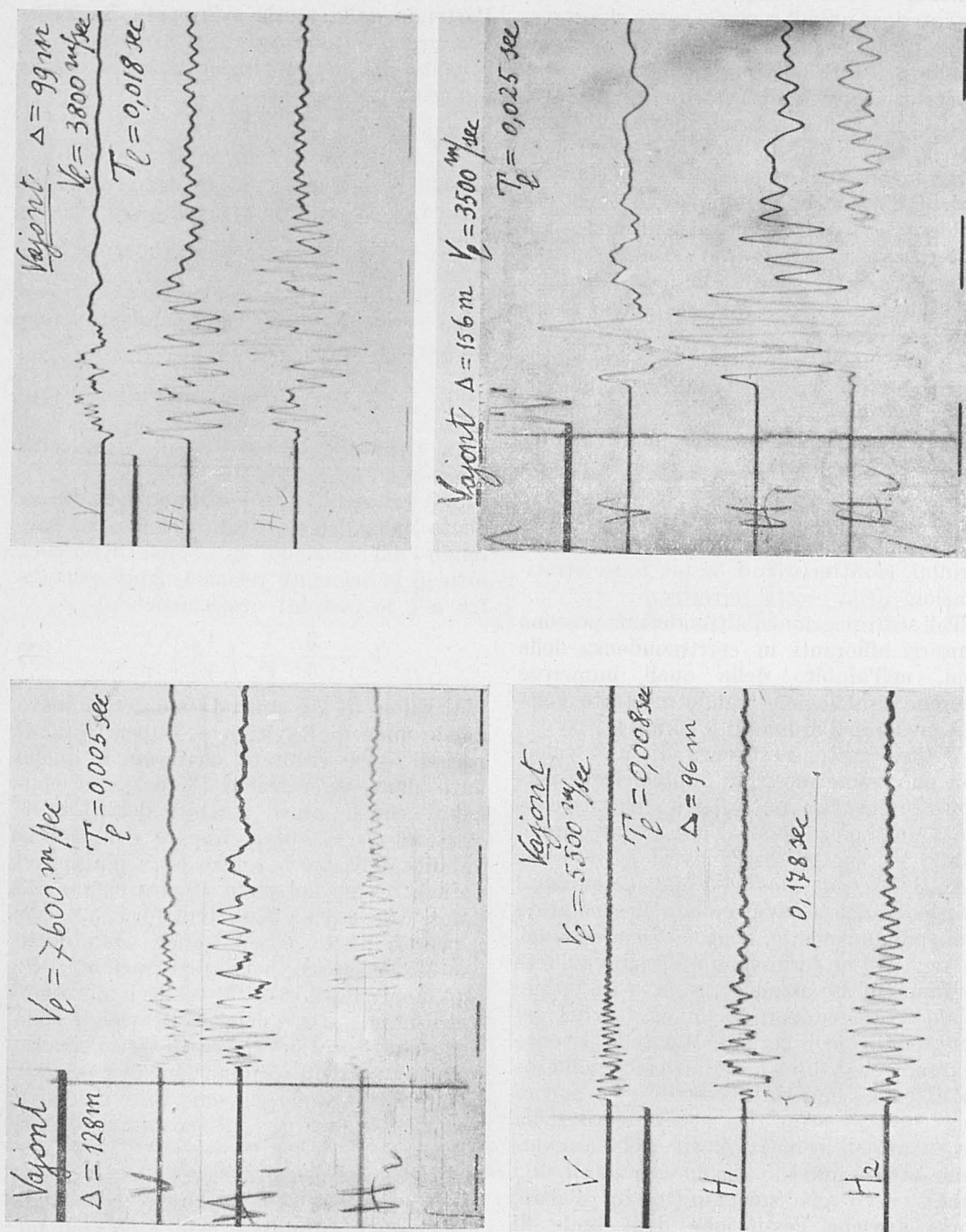
Fig. 4. - Dispersion nella stretta del Vajont, dal fondo valle al margine superiore.
